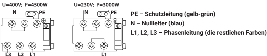
Abb. 2 - Etikette mit dem Schaltplan
