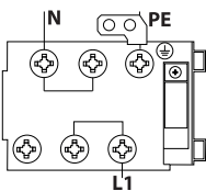
Obr. 2 - Štítek se schématem připojení
