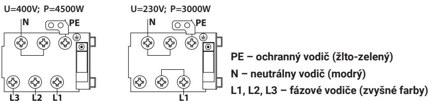
Obr. 2 – Schéma zapojenia
