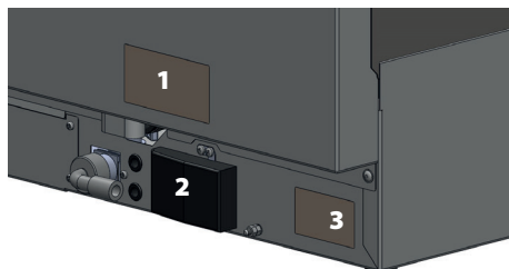
Obr. 3 – 1. Štítek se schématem zapojení; 2. Svorkovnicová skříň; 3. Štítek s údaji o spotřebiči
