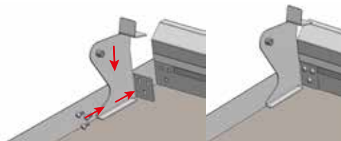
Rysunek 14. Montaż lewego zawiasu pokrywy (po lewej) oraz płyta z przykręconym lewym zawiasem (po prawej).
