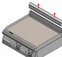
Bild 11. Demontage des Feuerschutzes.
