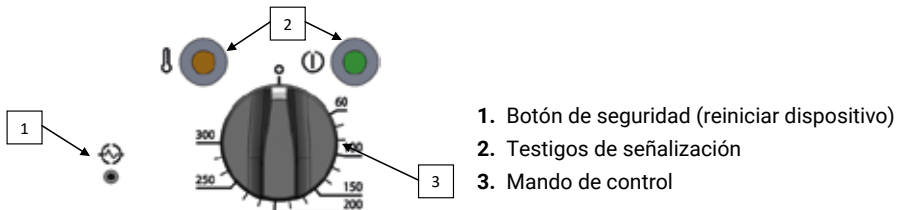
Figura 16. Elementos de control del dispositivo
