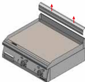
Obrázek č. 11. Demontáž zadního krytu.
