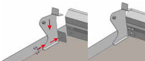
Obrázek č. 14. Montáž levého pantu víka (vlevo) a deska s příšroubovaným levým pantem (vpravo).
