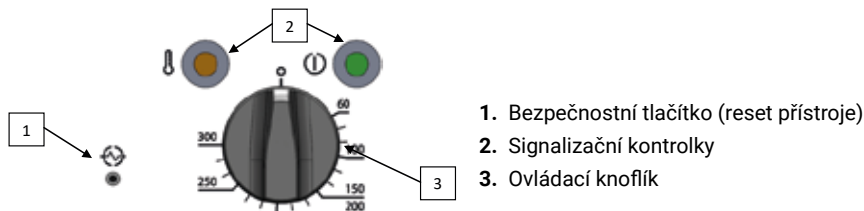
Obrázek č. 16. Řídicí prvky zařízení
