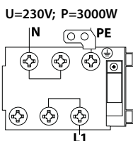
Obr. 2 - Štítek se schématem připojení
