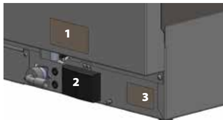
Rys. 3 – 1. Etykieta schematu podłączenia; 2. Skrzynka zaciskowa; 3. Tabliczka znamionowa
