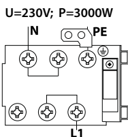
Obr. 2 – Schéma zapojenia
