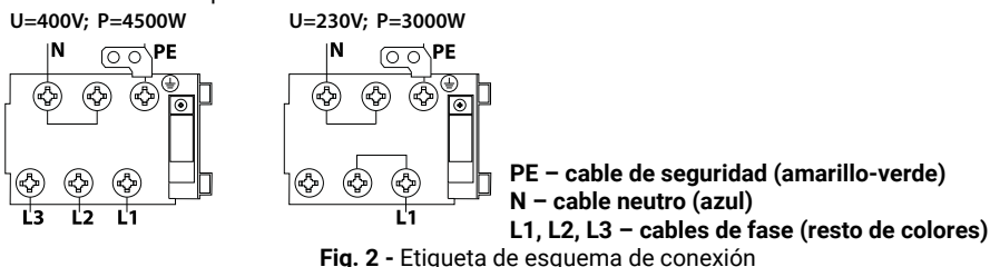
Fig. 2 - Etiqueta de esquema de conexión
